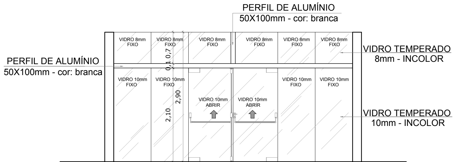
VISTA 1 ESC 1/50
