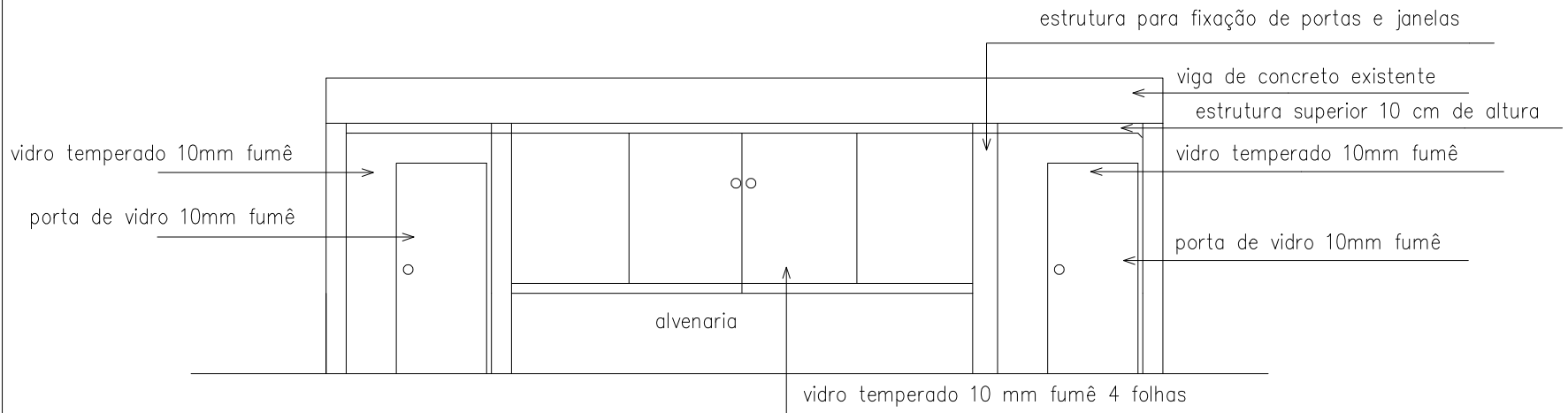
FACHADA FRENTE RUA
