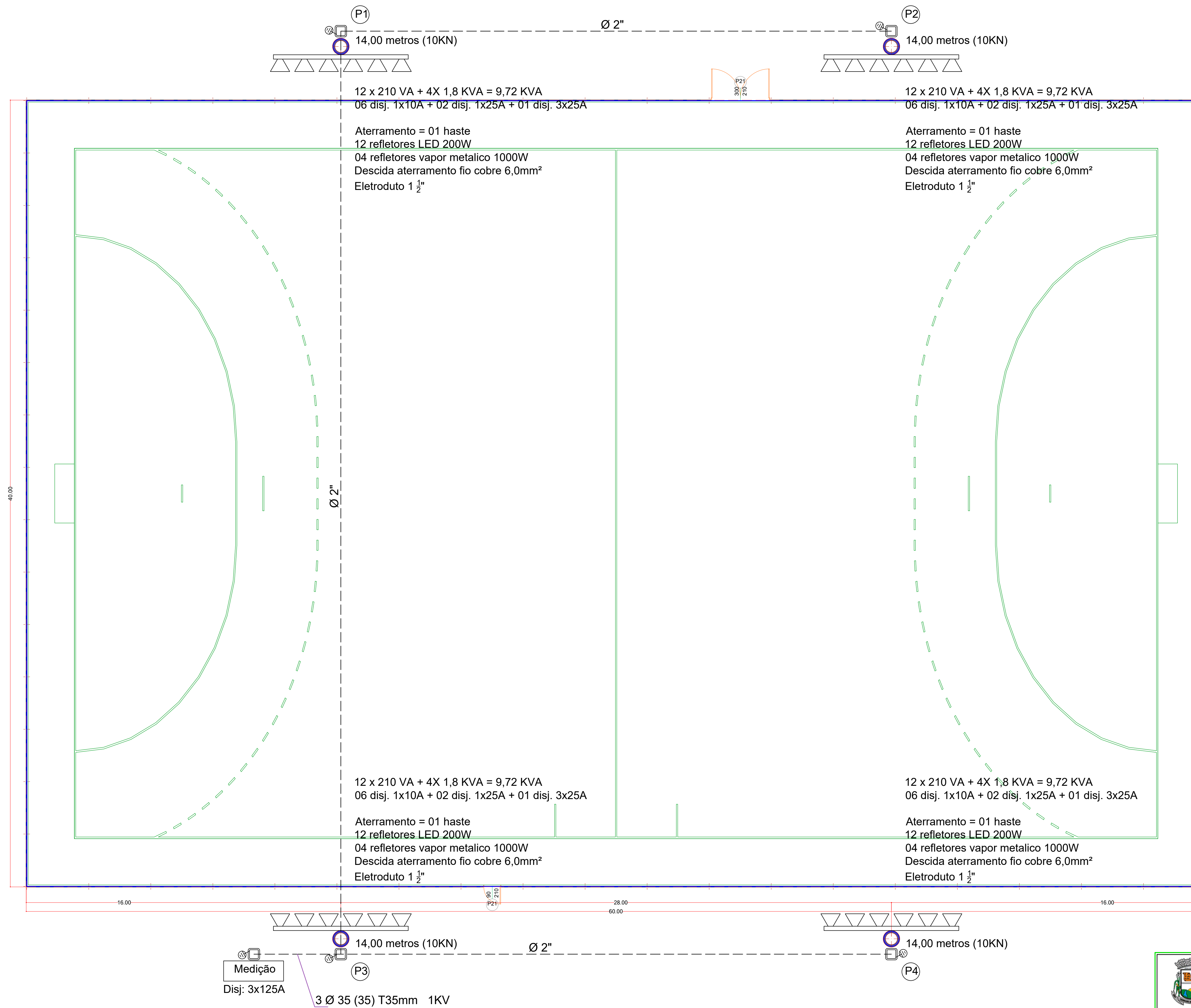
01 PLANTA BAIXA
