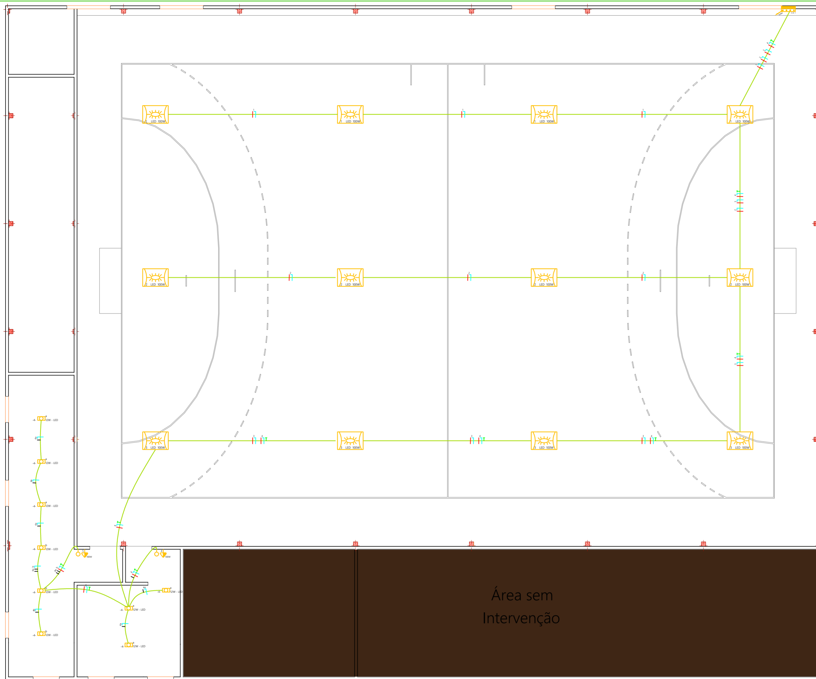
01 PLANTA BAIXA Projeto Elétrico
