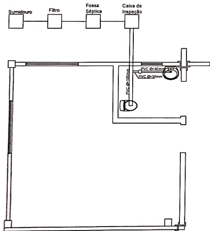
Projeto Hidrossanitário Escala: 1/50
