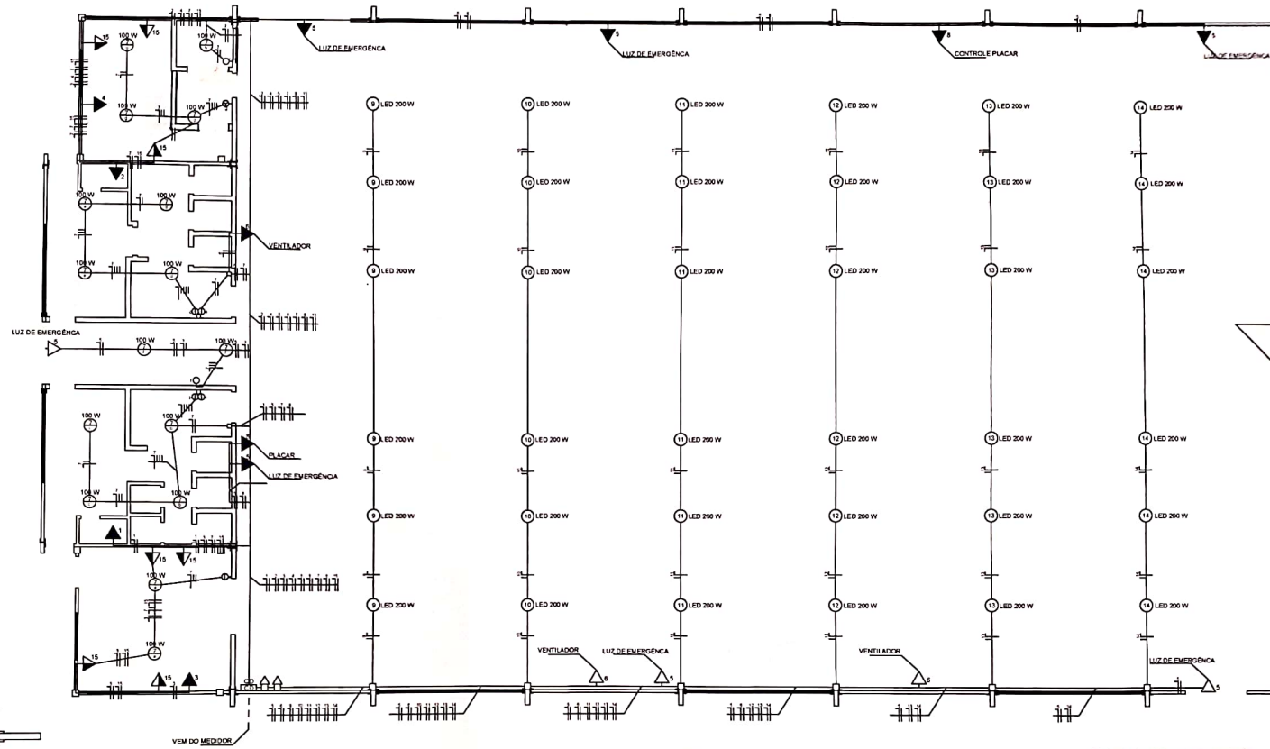
Projeto Elétrico Escala: 1/100
